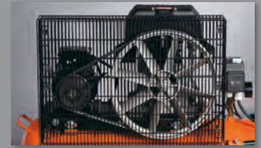
Keilriemenantrieb
